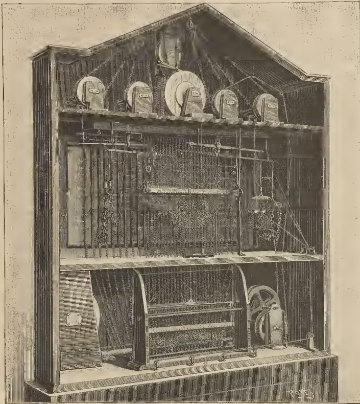
Fig. 2. — Mecanismo interior del diagraphómetro
